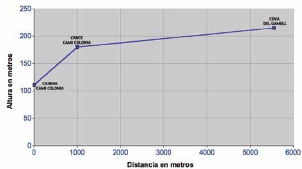
PERFIL RUTA 12
